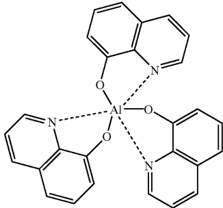
Alq3
