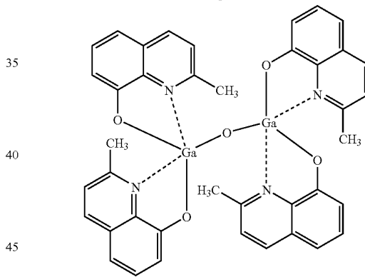
2(Gaq'2)
