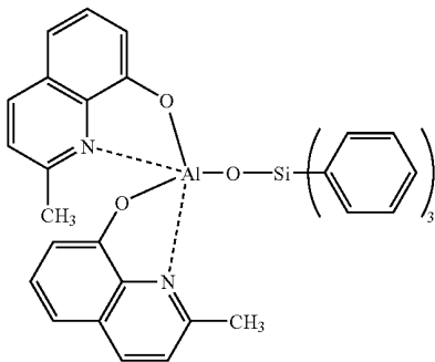
SALq
