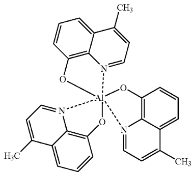
Almq3
