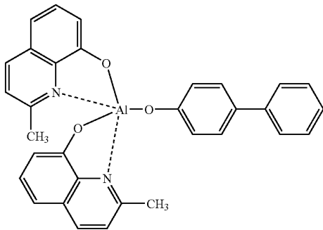
BAlq
